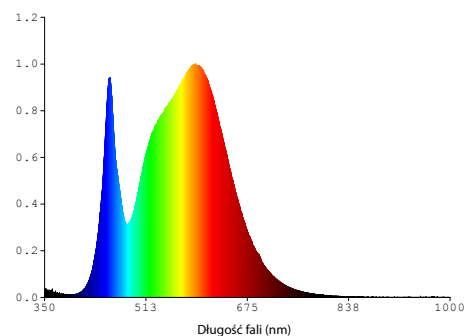
LEDSTAR ECO A65, 20W, NB - 4000K
